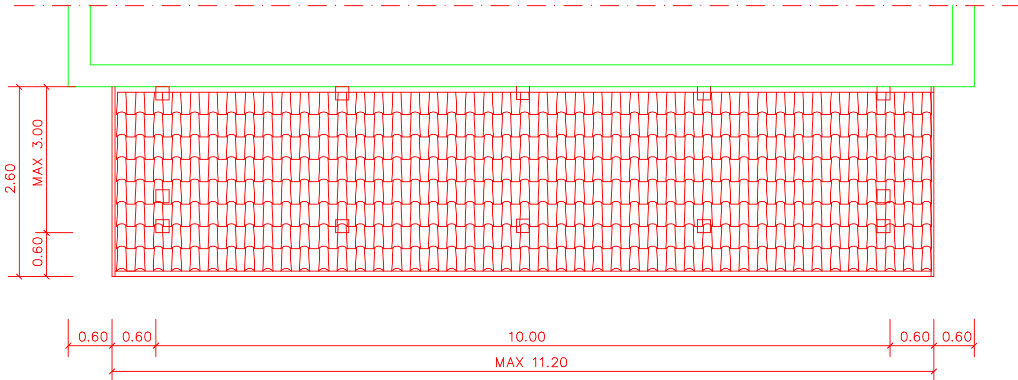
PIANTA DEL TETTO
