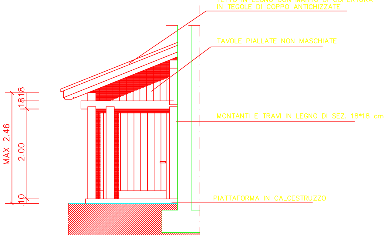
PROSPETTO FRONTALE
