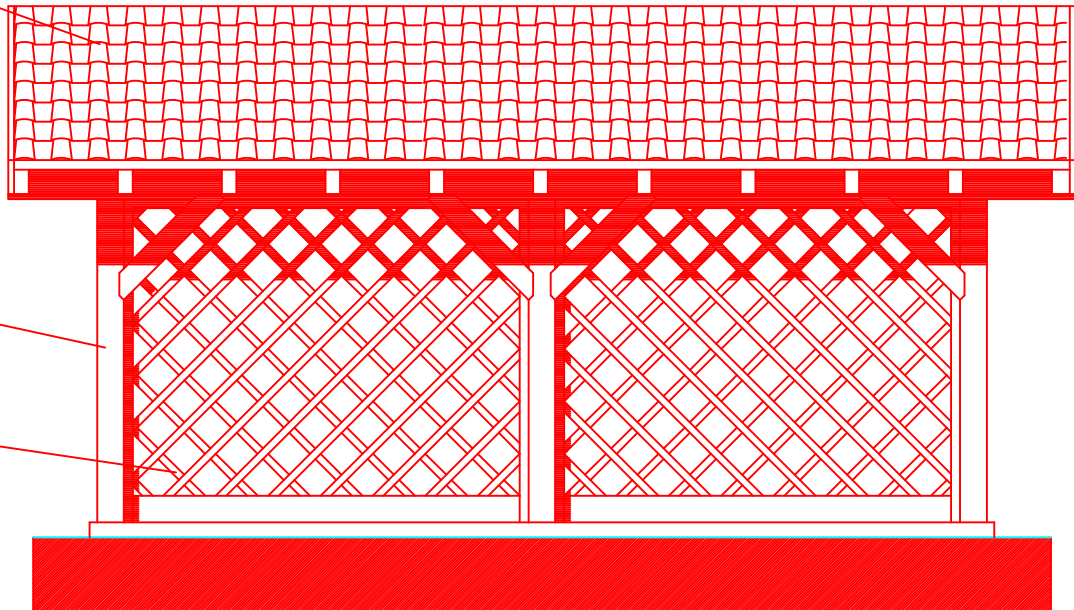
PROSPETTO LATERALE
