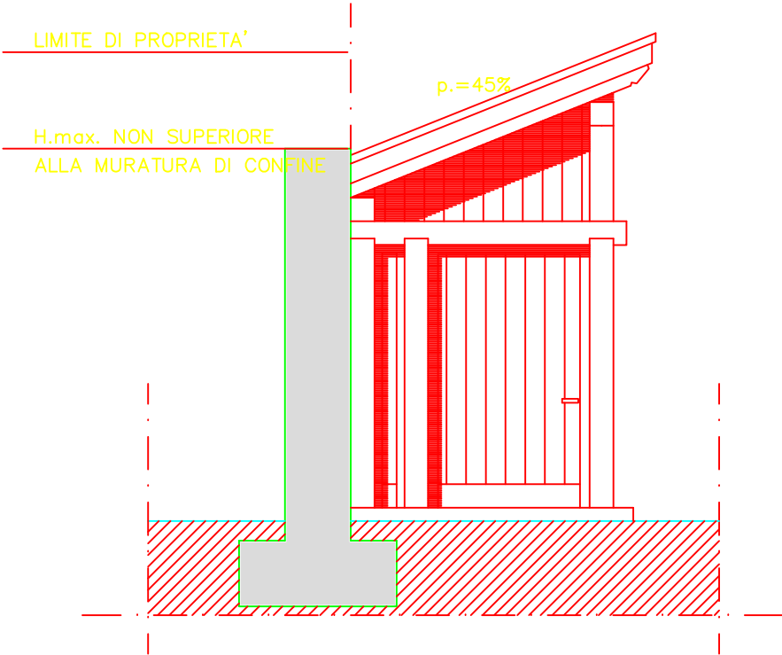
PROSPETTO FRONTALE
